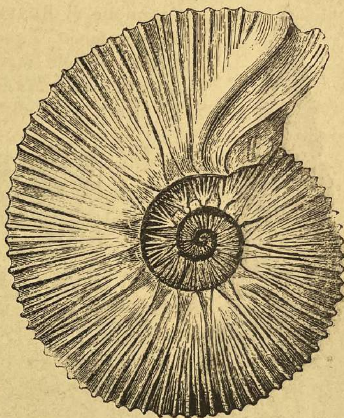
Fig. 333. — Olcostephanus astierianus d'Orb.
