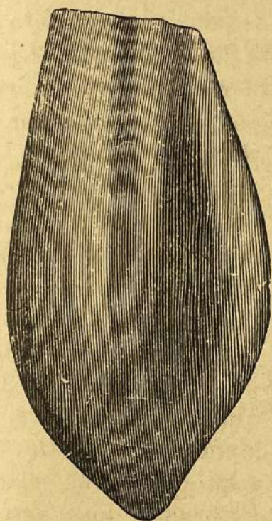
Fig. 332. — Duvalia dilatata Blainv.
