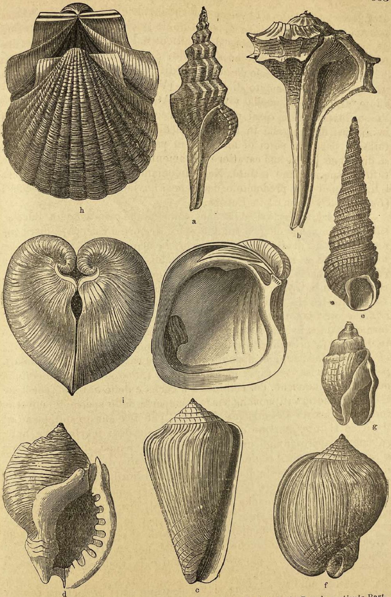
Fig. 365. — Alcuni molluschi miocenici. — a. Fusus longirostris Brocc., b. Pyrula rusticula Bast., c. Conus ponderosus Brocc., d. Ranella marginata Brocc., e. Turritella turris Bast., f. Cassis saburon Lam., g. Melanopsis Martiniana Fér., h. Pecten aduncus Eichw., i. Dreissensia conglobata Partsch.
