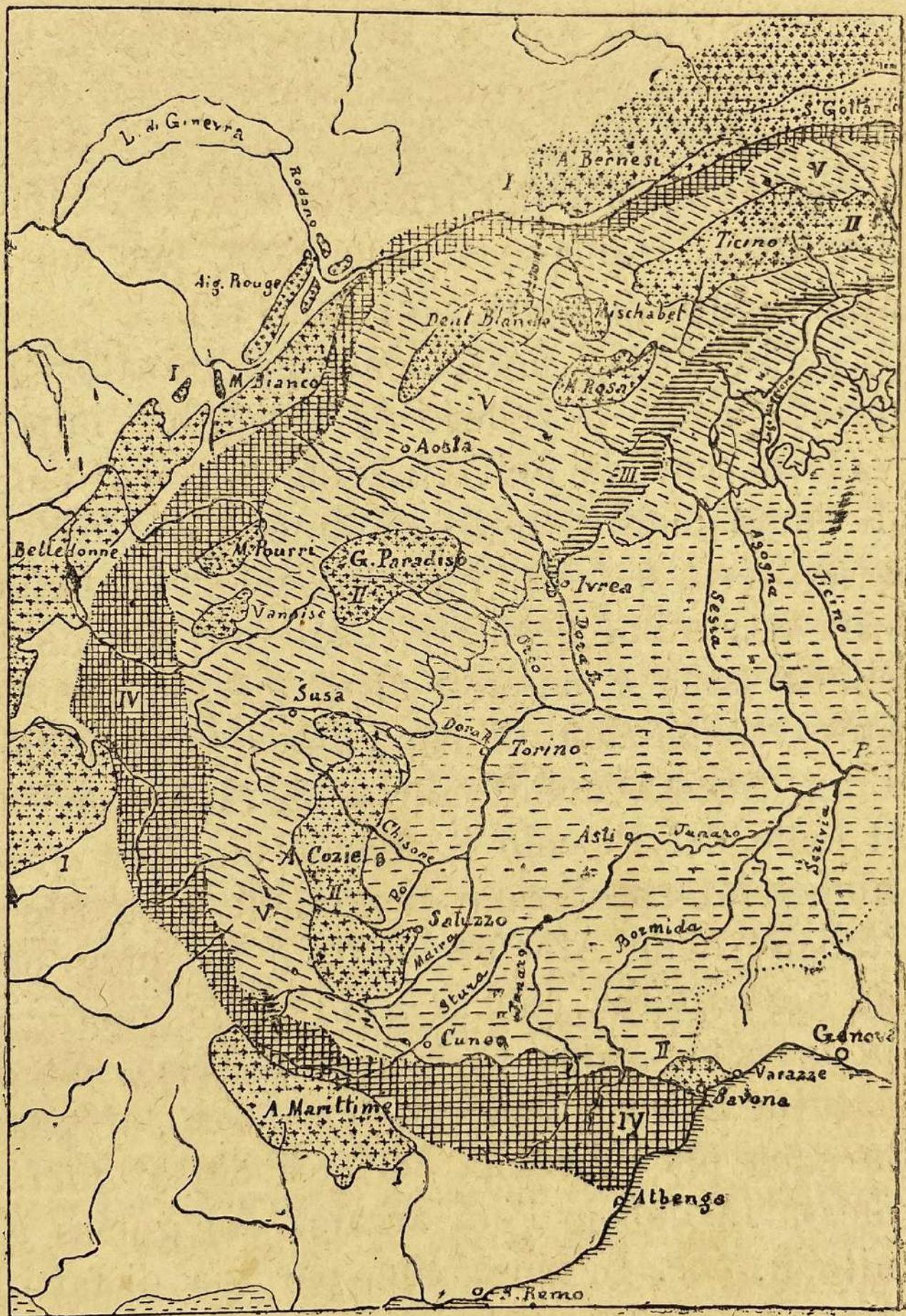
Fig. 150. — Schizzo delle zone orotettoniche delle Alpi Occidentali, secondo DIENER e NOVARESE.
