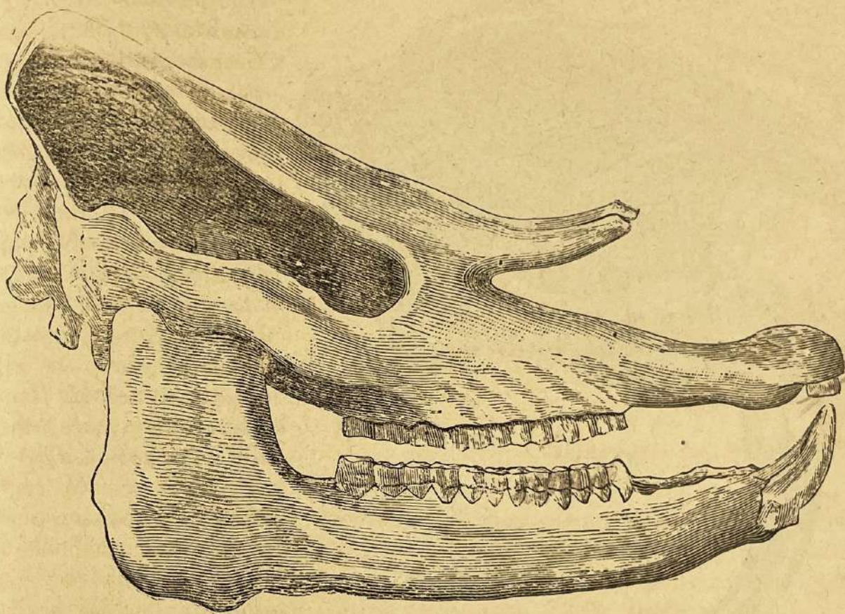
Fig. 367. — Rhinoceros ( Aceratherium ) incisivus Cuv. (gr. 1/6).
